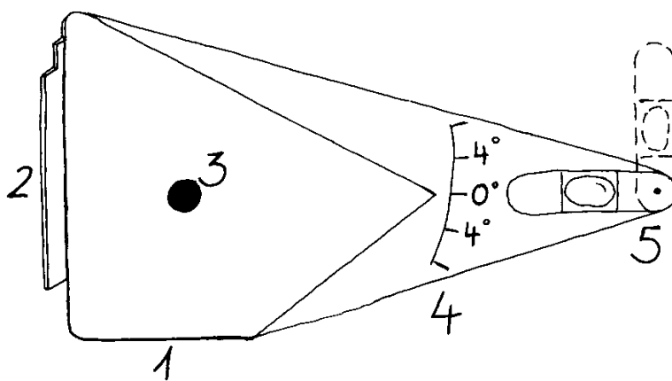
Abbildung 2-12: Anlagemessgerät
