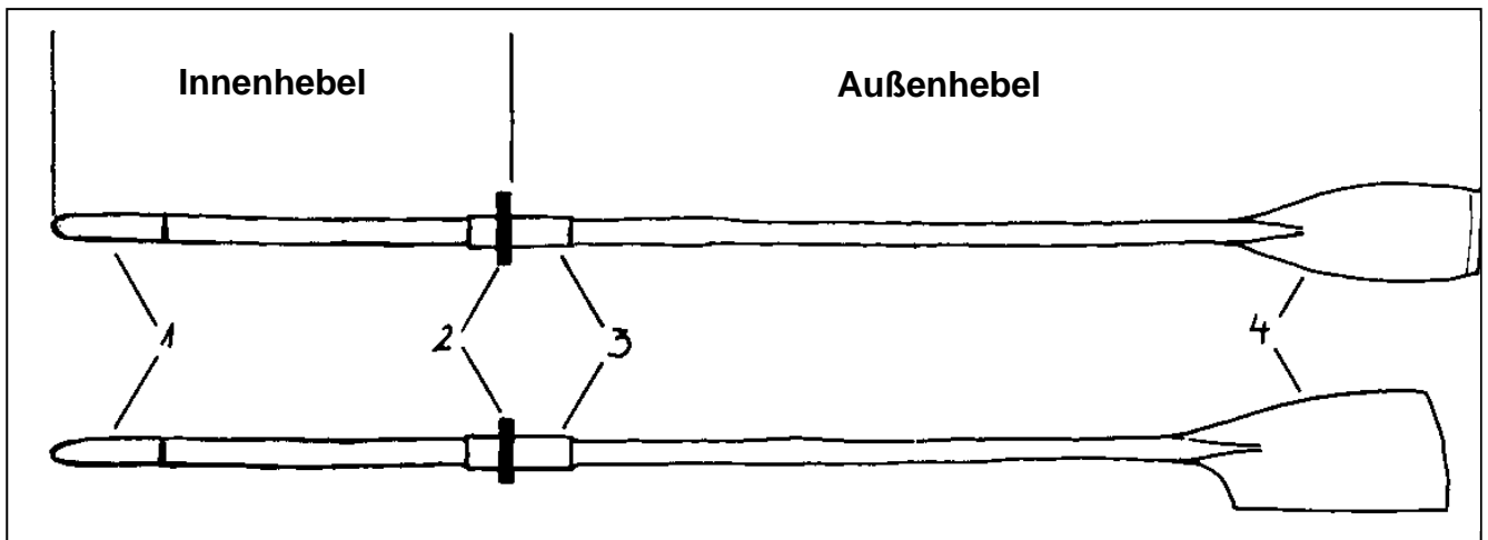
Abbildung 2-4: Bezeichnung der Teile am Skull (oben Macon-Blatt, unten Big-Blade):
