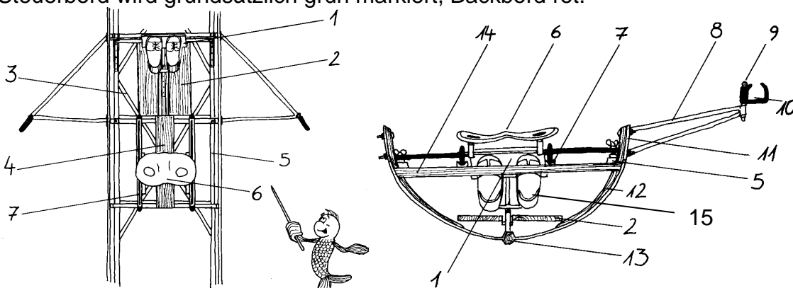
Abbildung 2-3: Bezeichnungen beim Ruderplatz (Aufsicht und Querschnitt)
