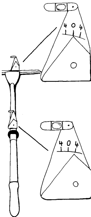
Abbildung 2-13: Messen der Anlage am Skull
